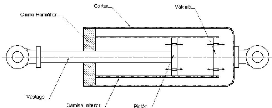
Esquema del amortiguador
